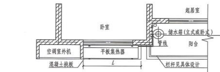
平面布置示意图
