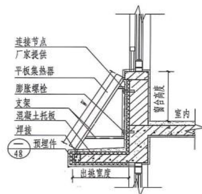
剖面布置示意图一 (低窗台)
