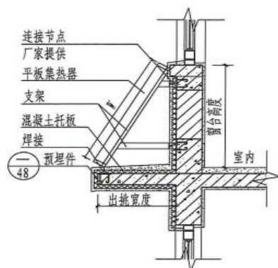
剖面布置示意图二 (900mm高窗台)
